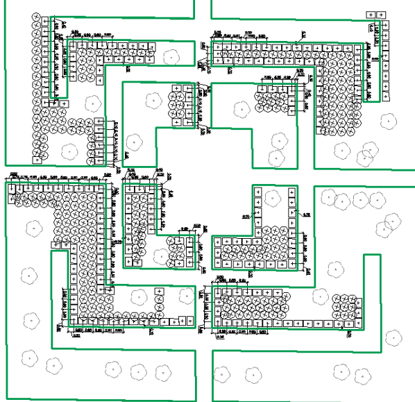
WYMIAROWANIE DOCEŁOWEGO OBRYSU ZYWOPLÓTÓW SKALA 1:200
