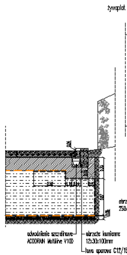
Nawierzchnia z płyt kamiennych
