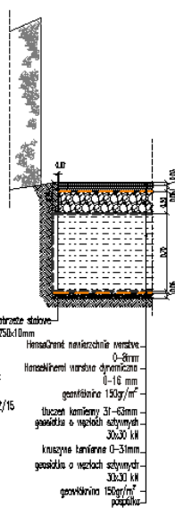
Nawierzchnia żwirowa (HanseGrand)
